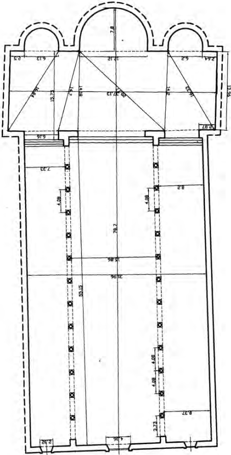
5) Plan de la cathédrale de Salerne entre la fin du XI e et le début du XII e siècle (BRACA, 2011)
